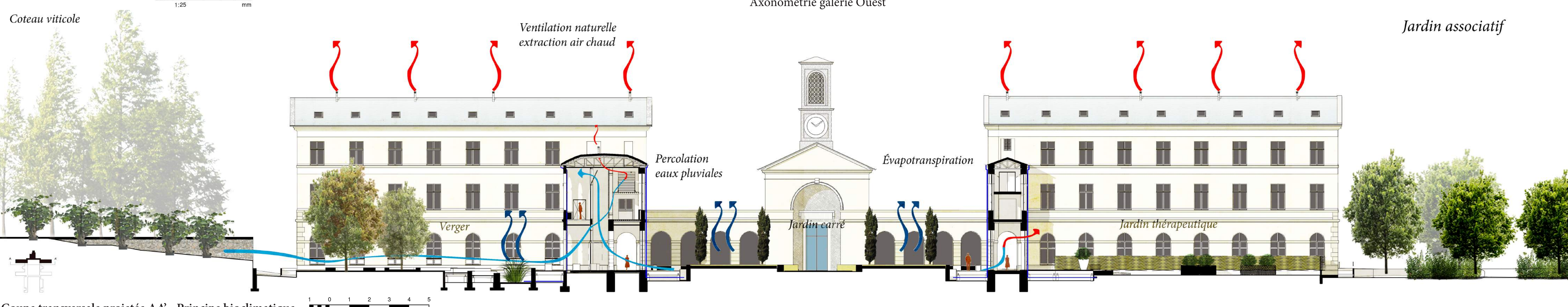
Coupe transversale projetée AA' - Principe bioclimatique
