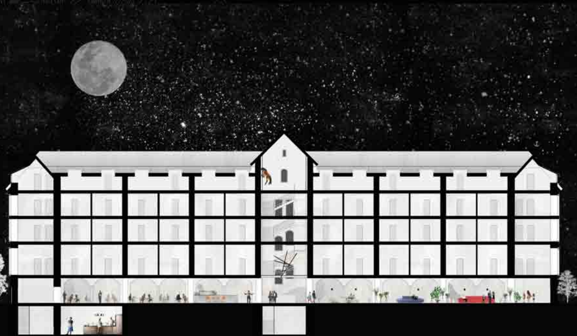
COUPE LONGITUDINALE 1/200
