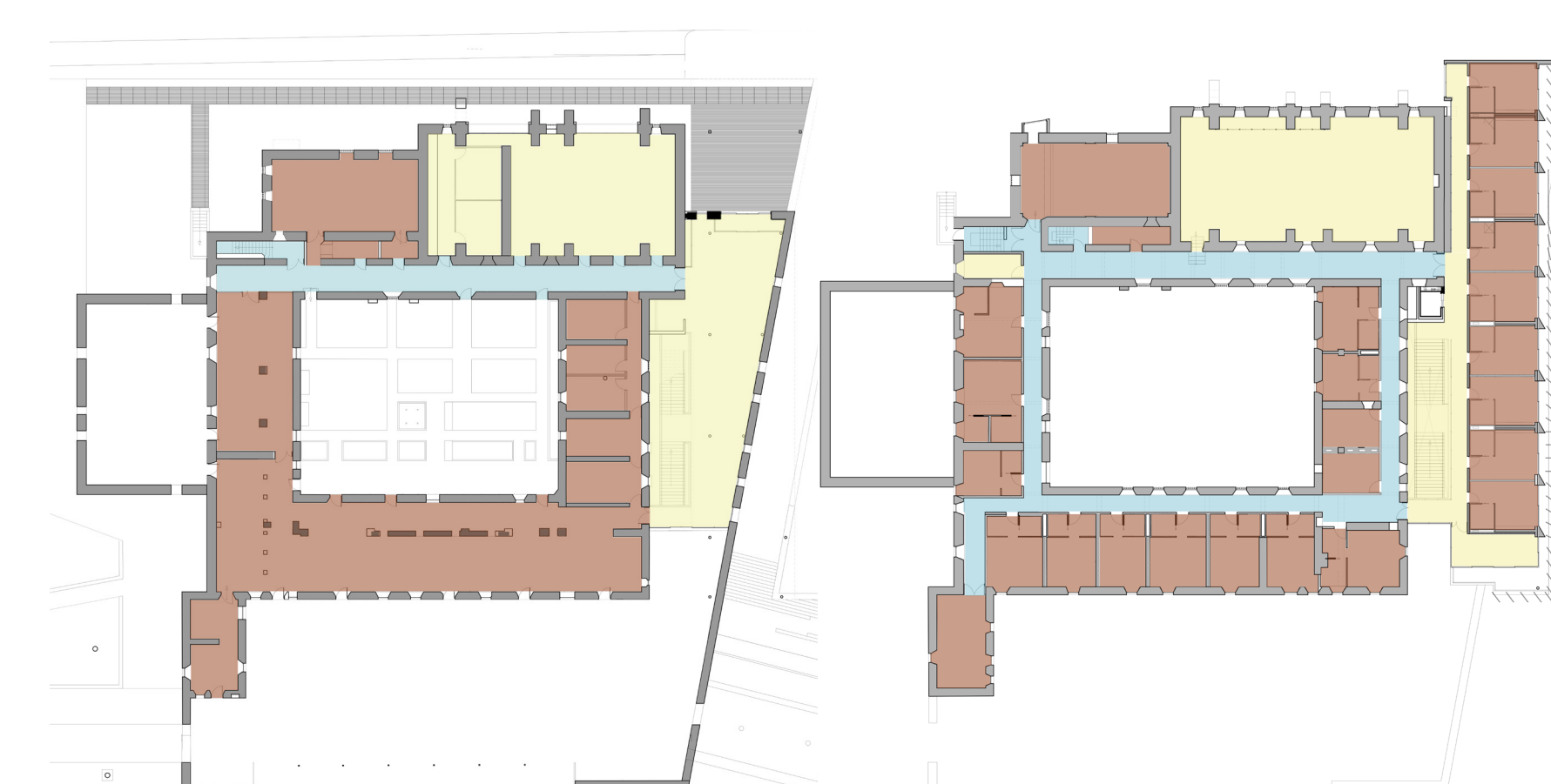
CHAUDS TEMPÉRÉS FRAÏS THERMIQUE ET CIRCULATION AU RDC THERMIQUE ET CIRCULATION AU R+1
