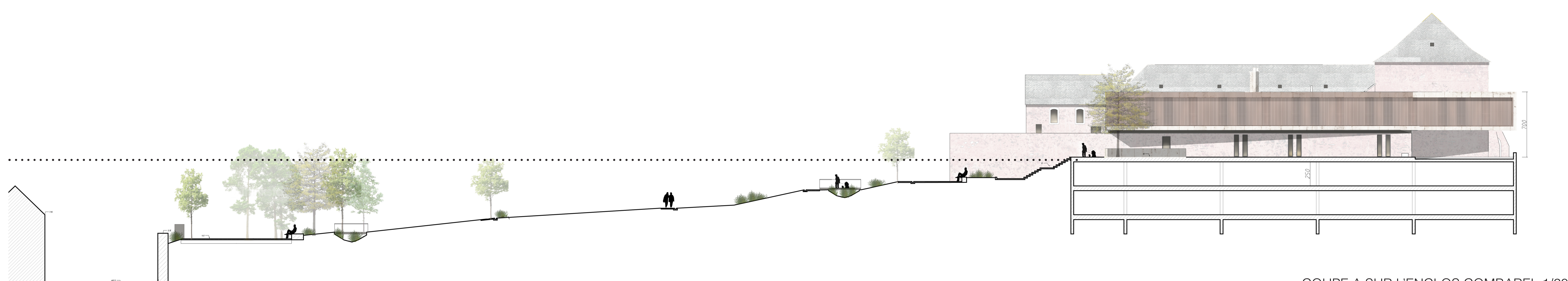
COUPE A SUR L'ENCLOS COMBAREL 1/200
