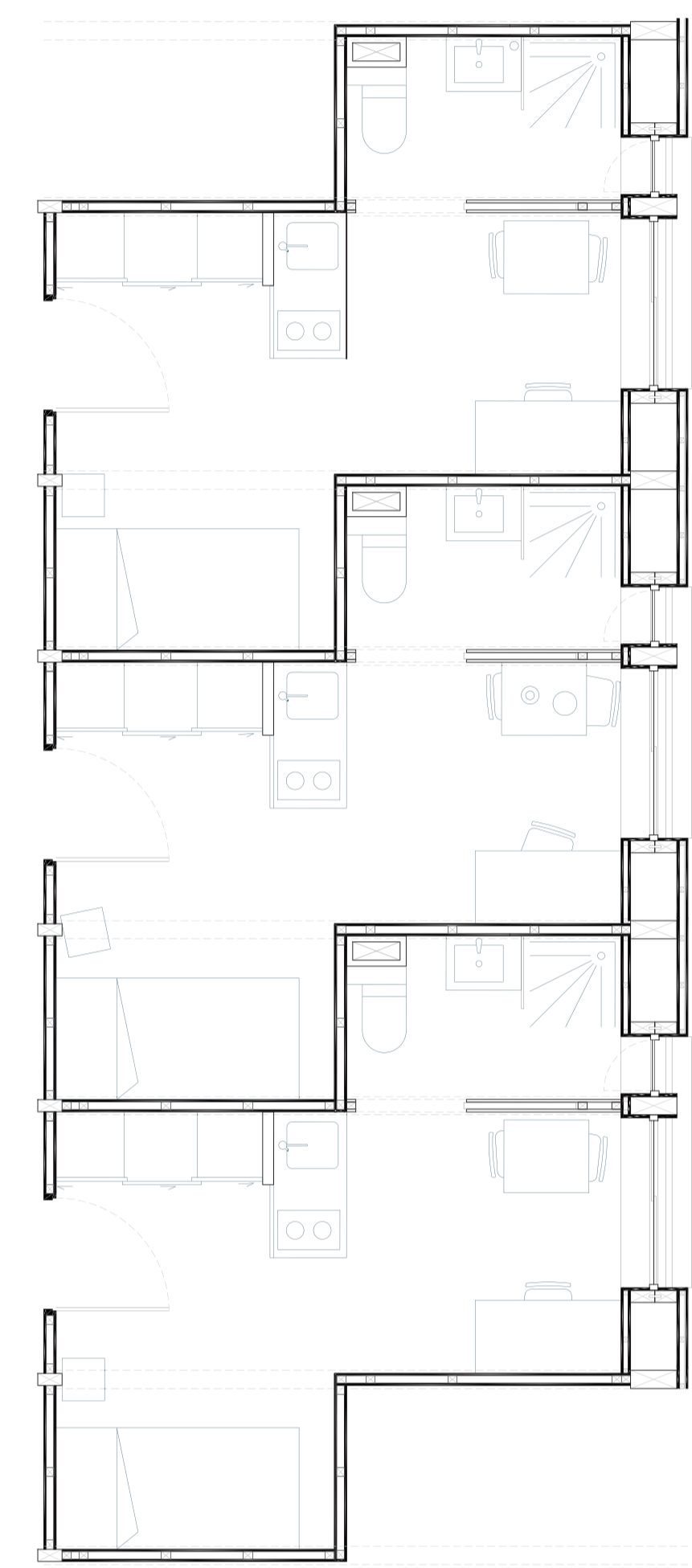
Typologie des Logements 1:50°
