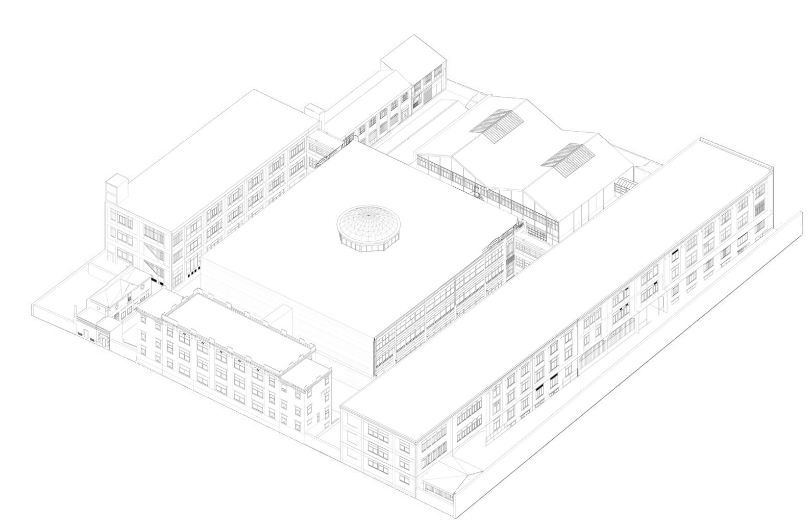
Axonométrie du site existant
