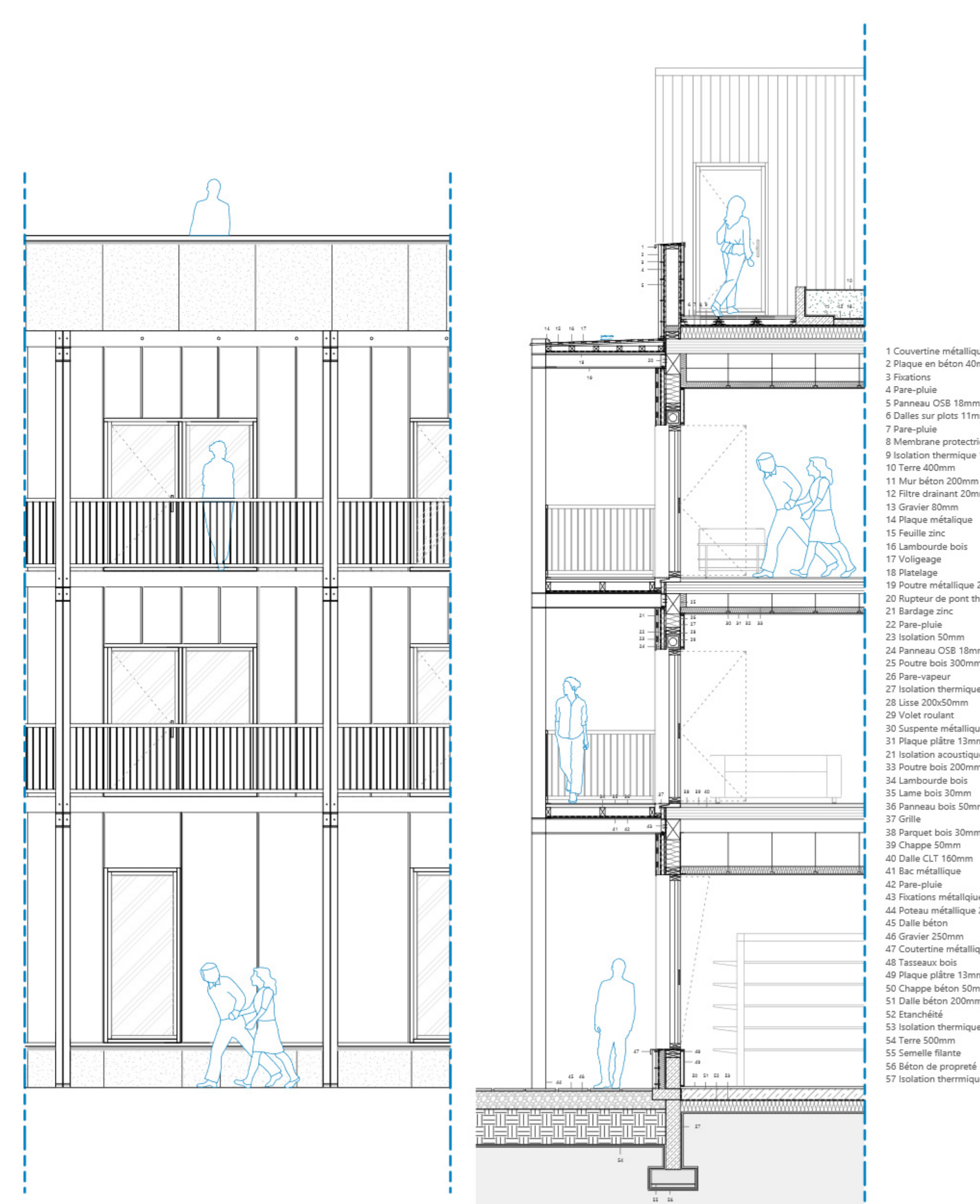
Détails 1/50
