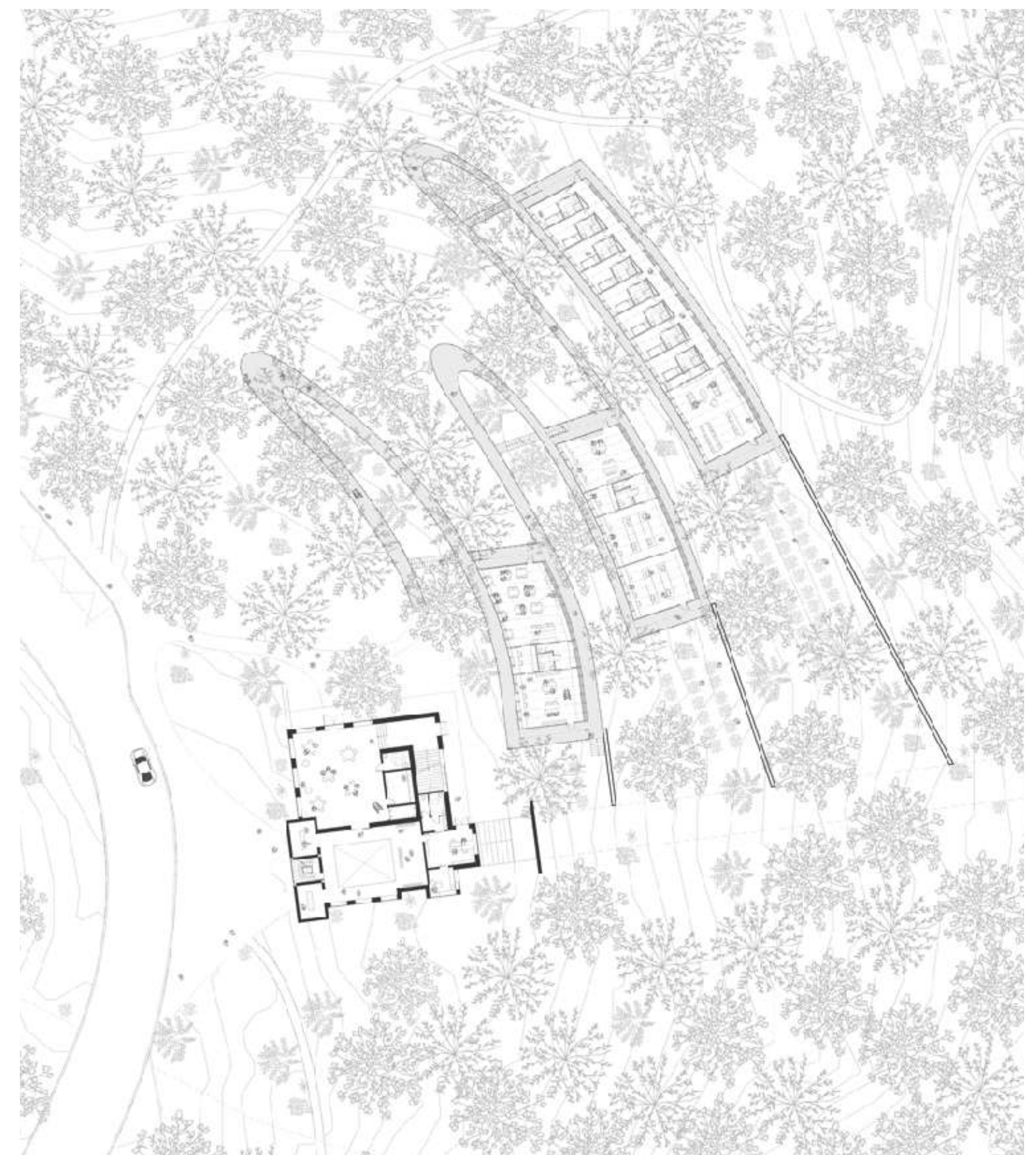
PLAN D'ENSEMBLE
