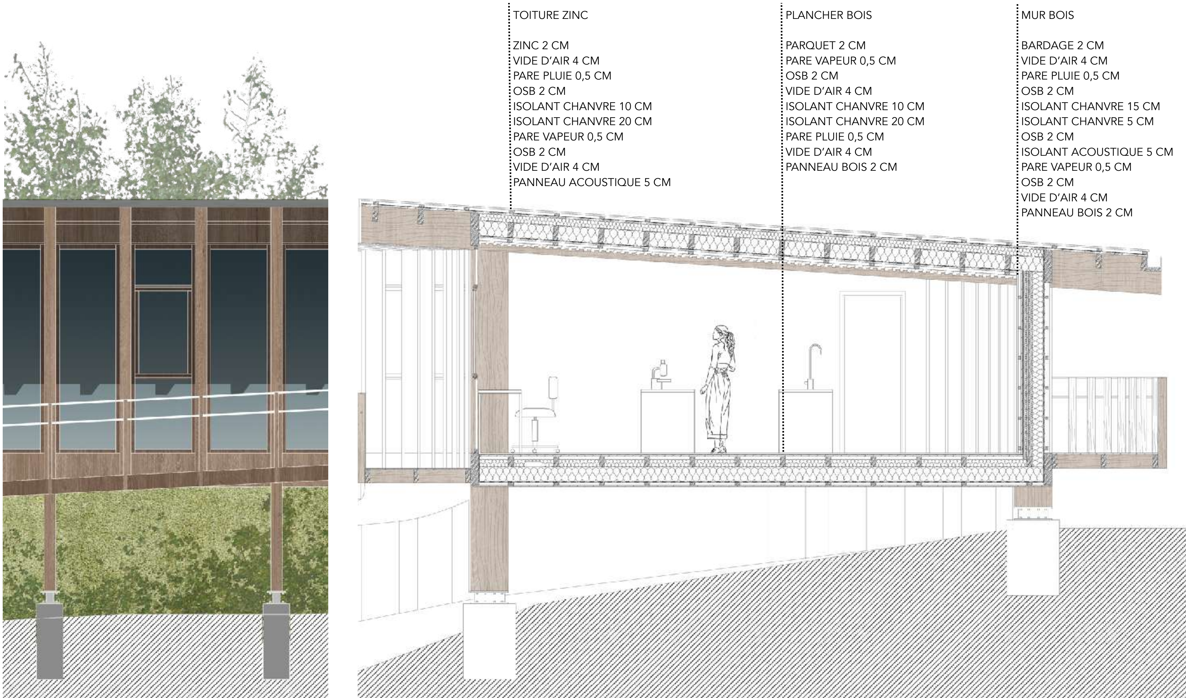
ÉLÉVATION
