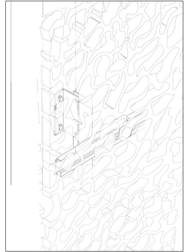
Axonométrie structurelle
