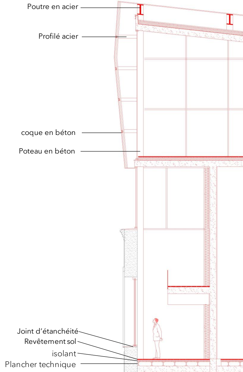
Coupe structurelle
