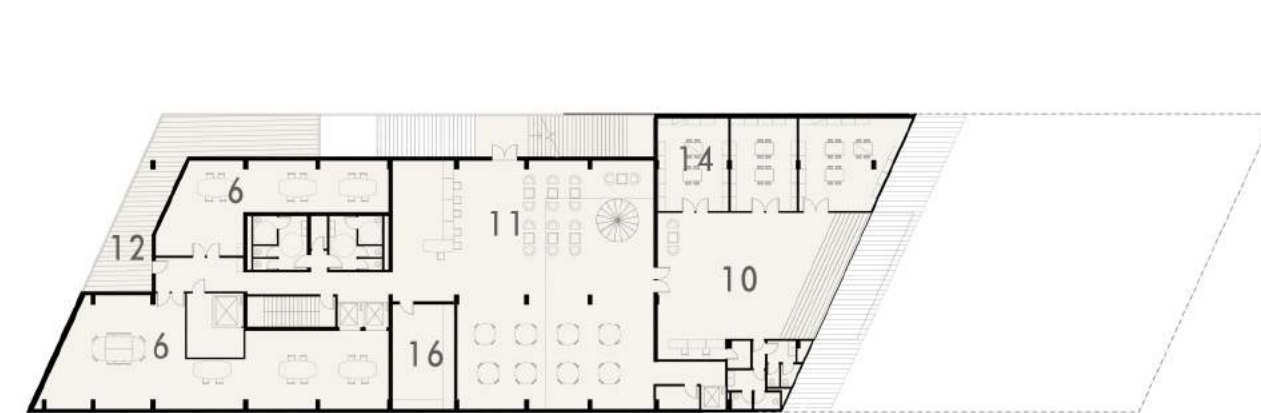
R+4 (+ 19.00M)
