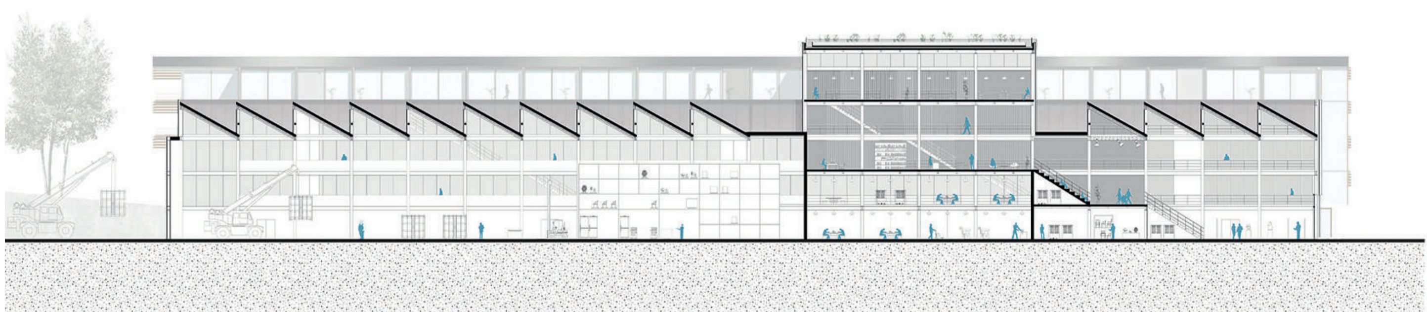
COUPE LONGITUDINALE BB'
