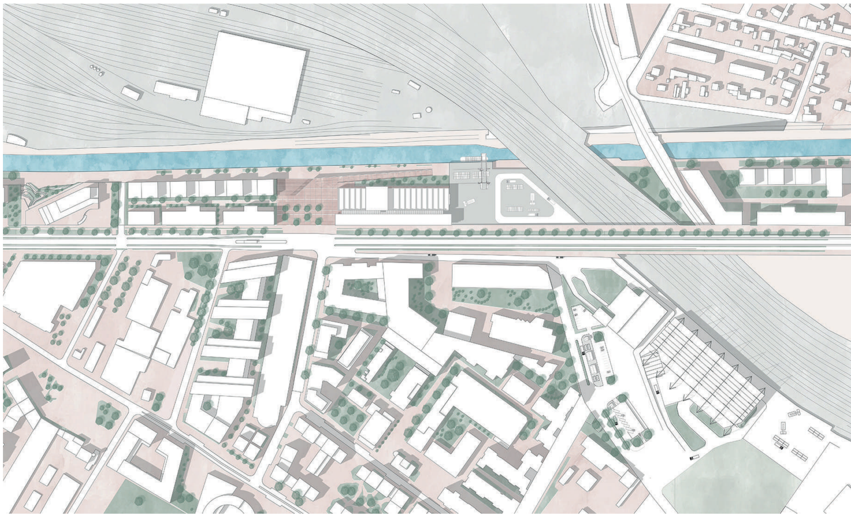
PLAN MASSE URBAIN
