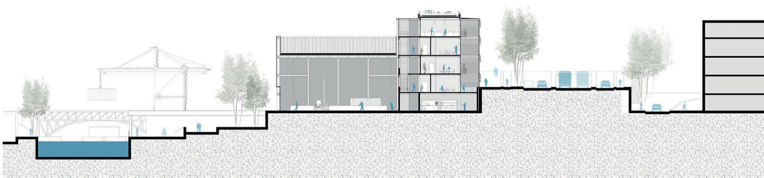
COUPE TRANSVERSALE AA'
