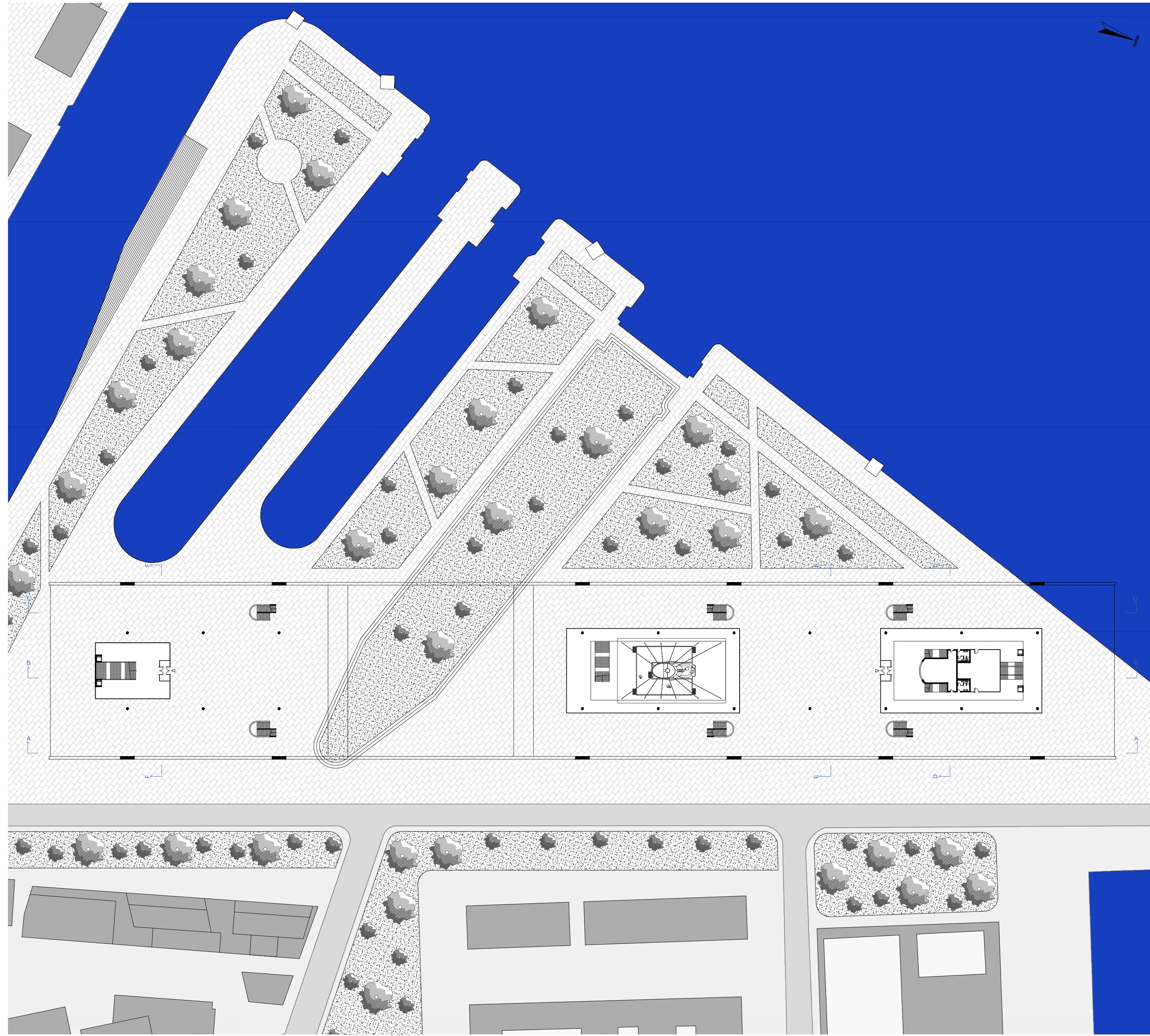
Plan RDC
