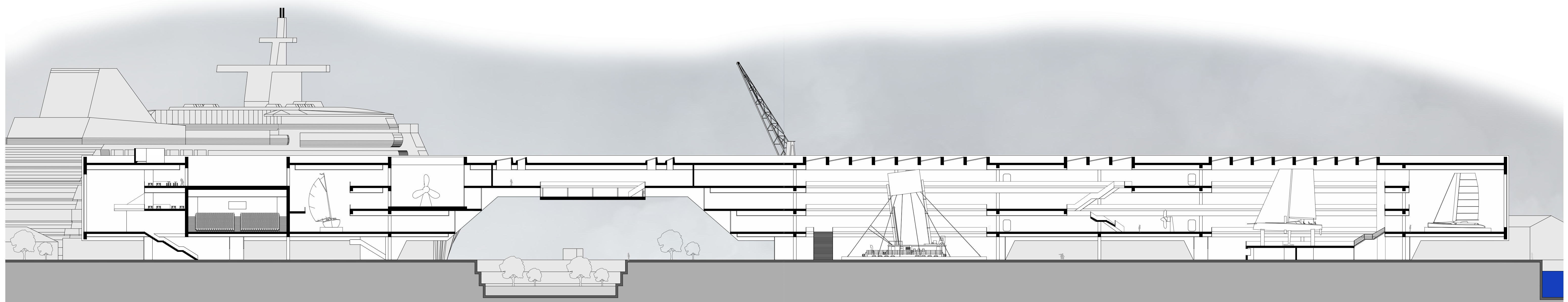
Coupe BB
