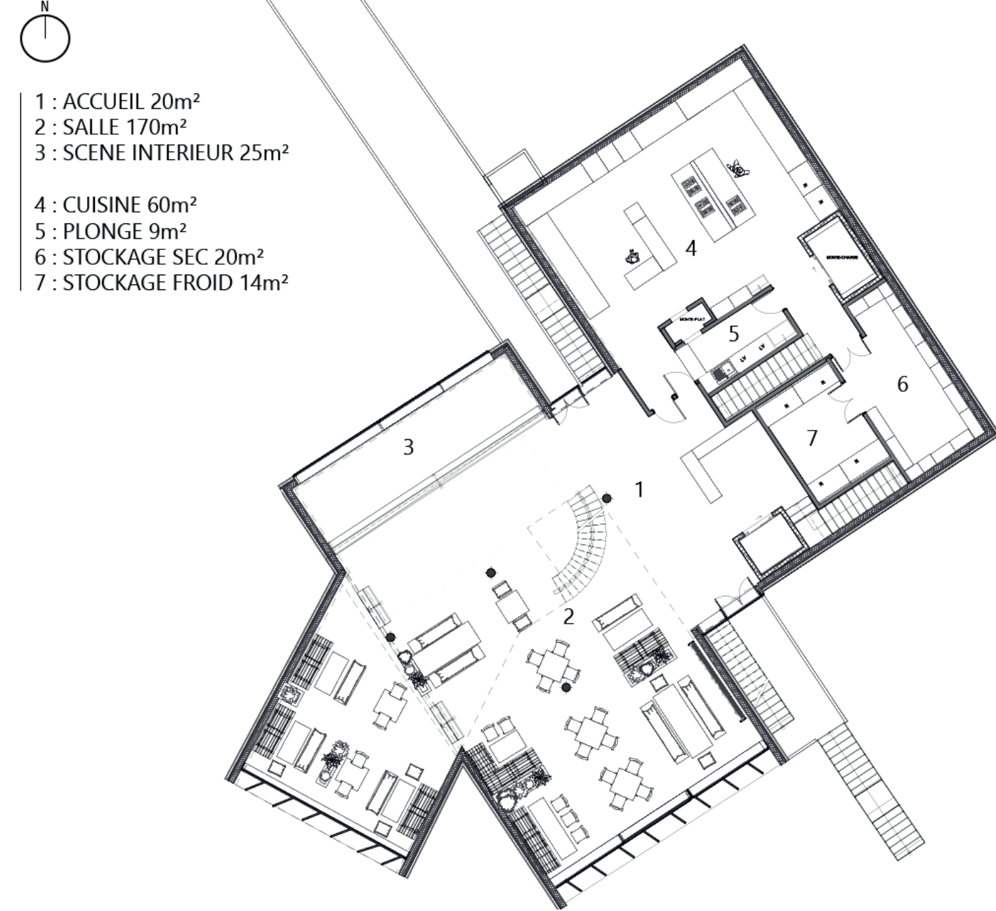
PLAN R+2
