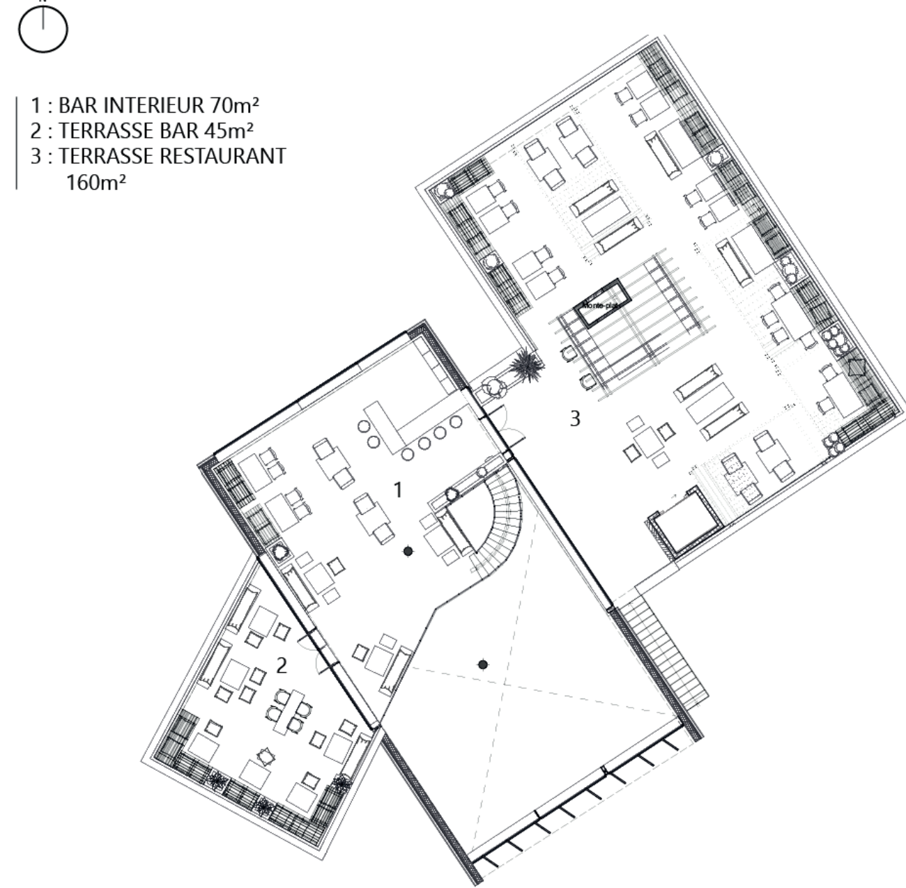
PLAN R+2
