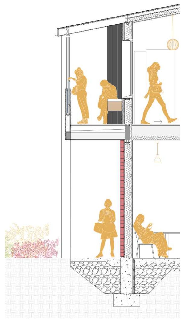
Coupe détail de coursives, 1:50
