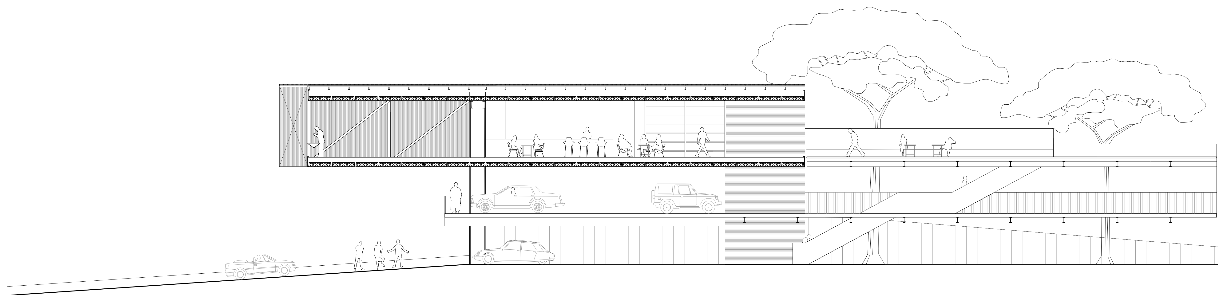
Coupe longitudinale du restaurant 1/100
