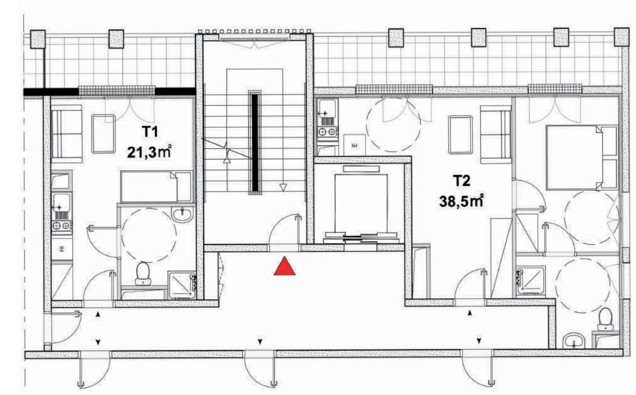
Extrait de plan R+4 résidence séniors 1/100
