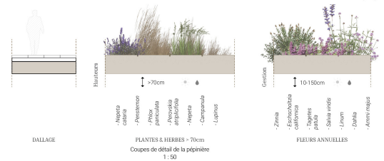
DALLAGE PLANTES & HERBES > 70cm Coupes de détail de la pépinière 1:50
