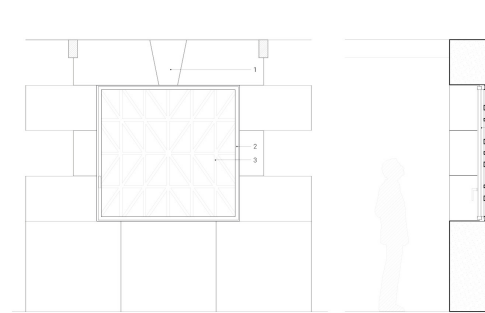
Détail claustra en pierre 1:20
