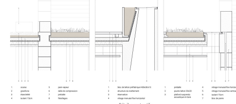
Détails constructifs 1:50
