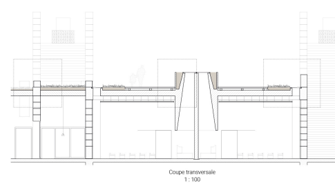
Coupe transversale 1:100
