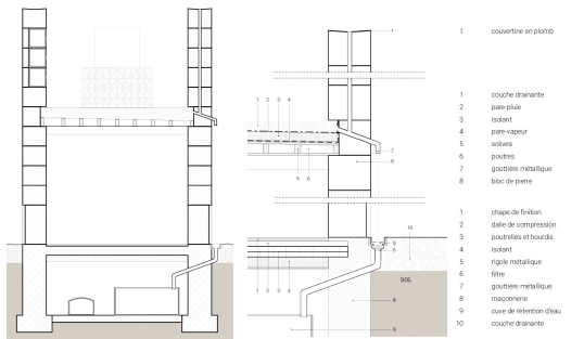
Coupe transversale 1:50 Détails constructifs 1:25
