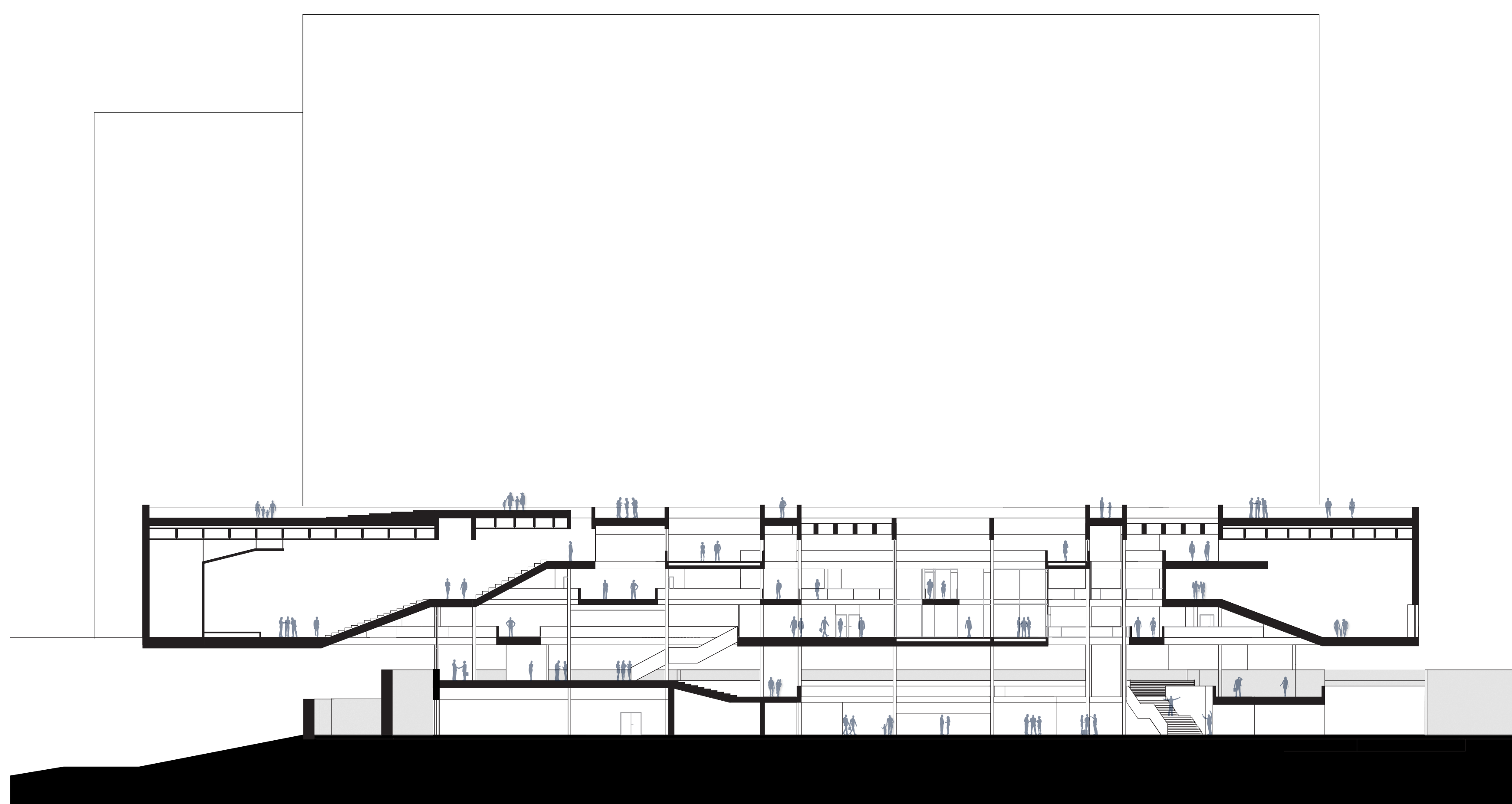
COUPE LONGITUDINALE DU CENTRE DE CONFÉRENCE
