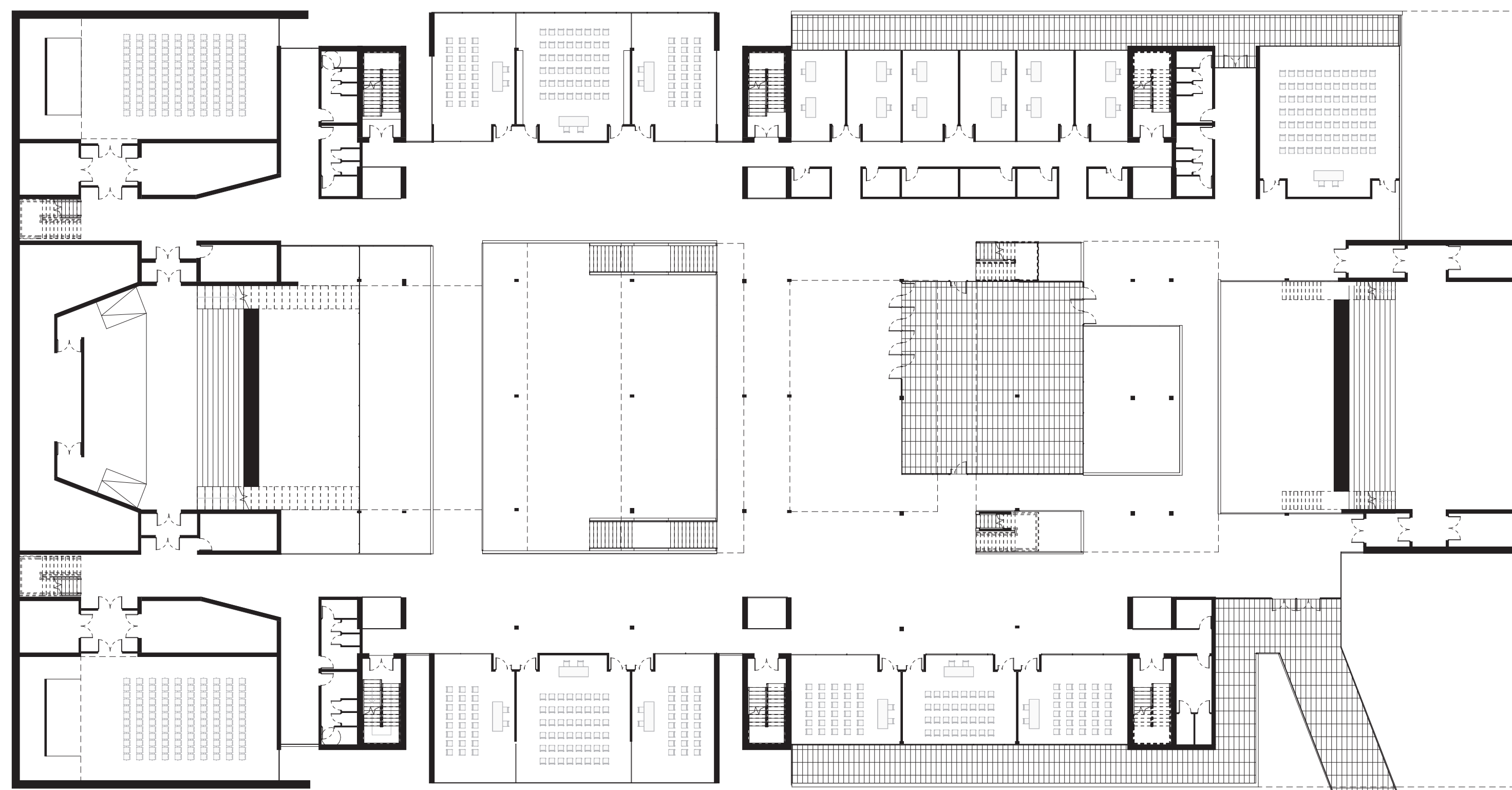
PLAN R+3 1.200 ème
