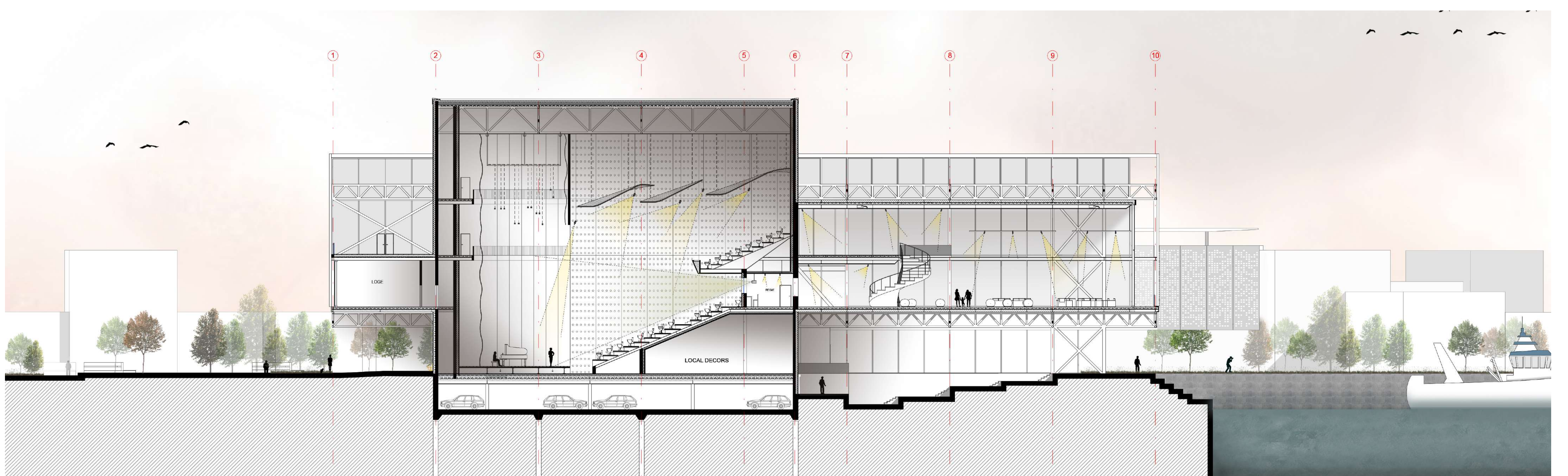
COUPE 1 ECH 1/200
