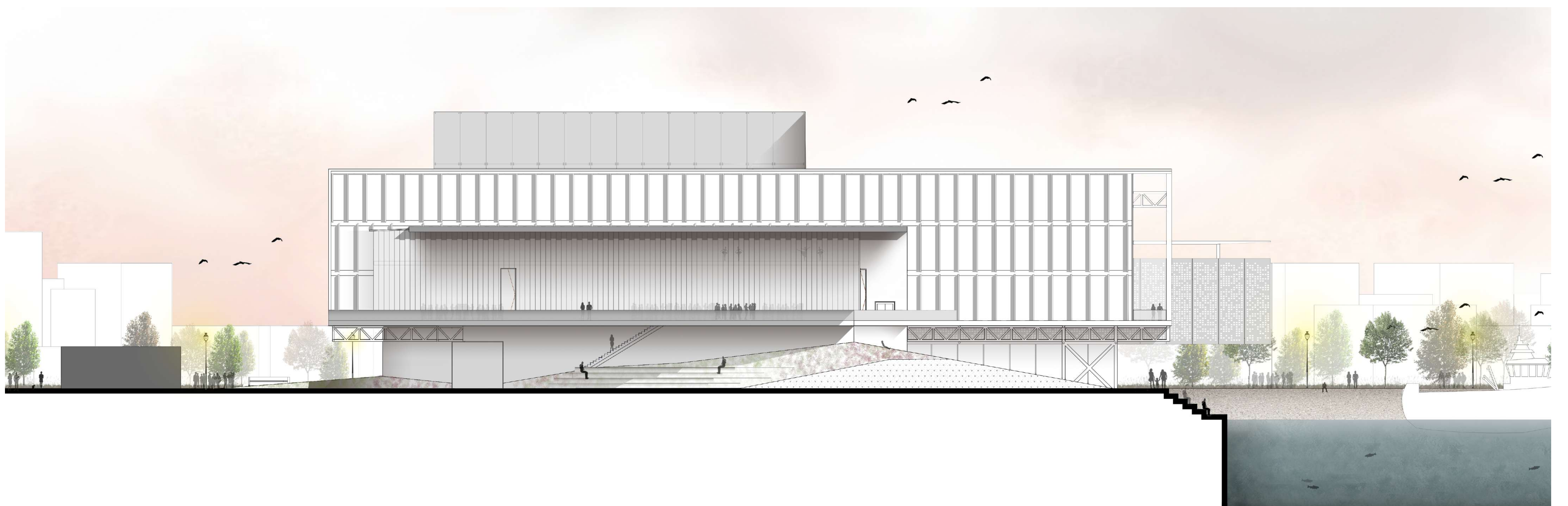
ÉLEVATION OUEST ECH 1/200
