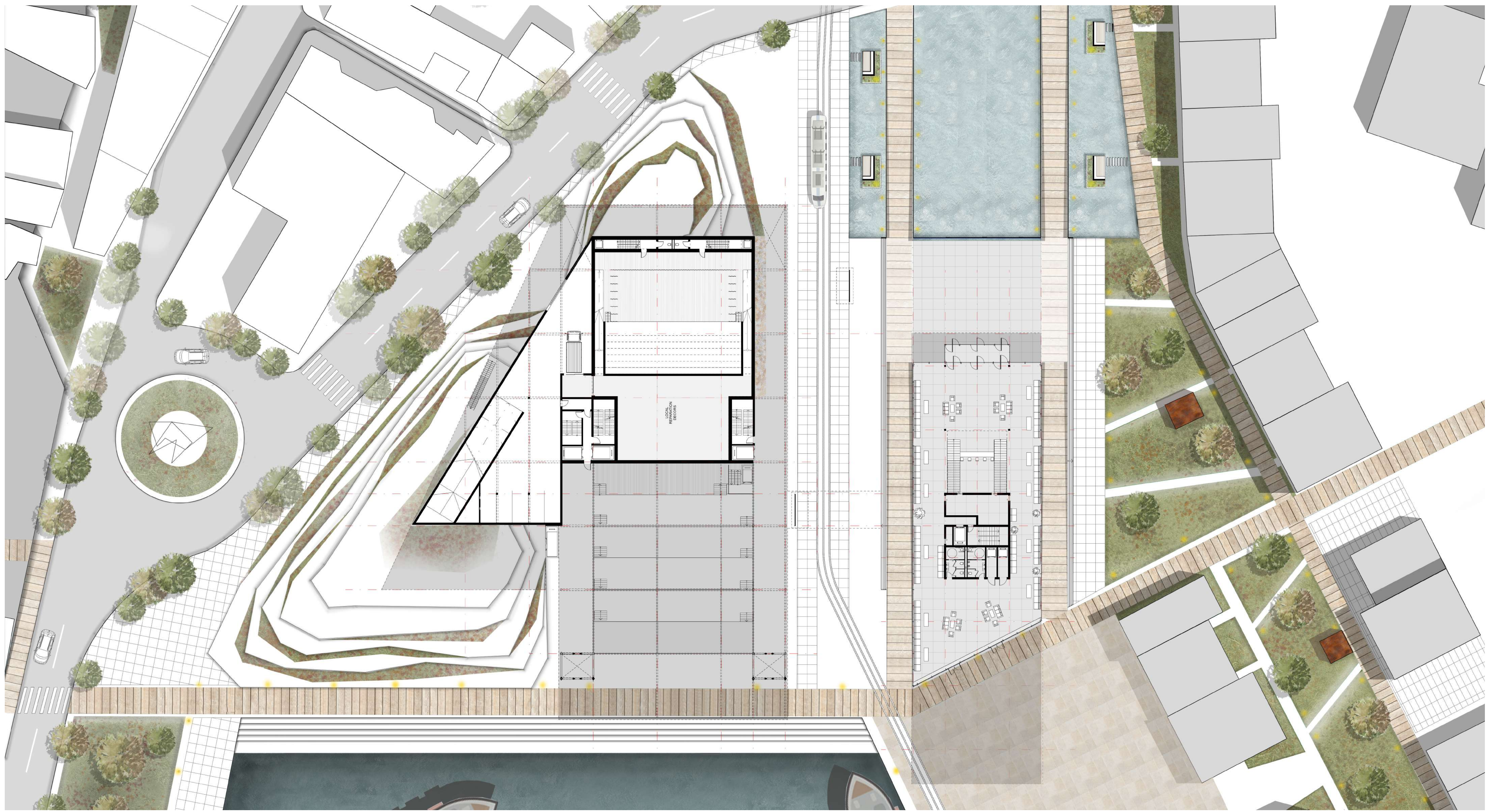
PLAN MASSE - RDC 0 10m 20m
