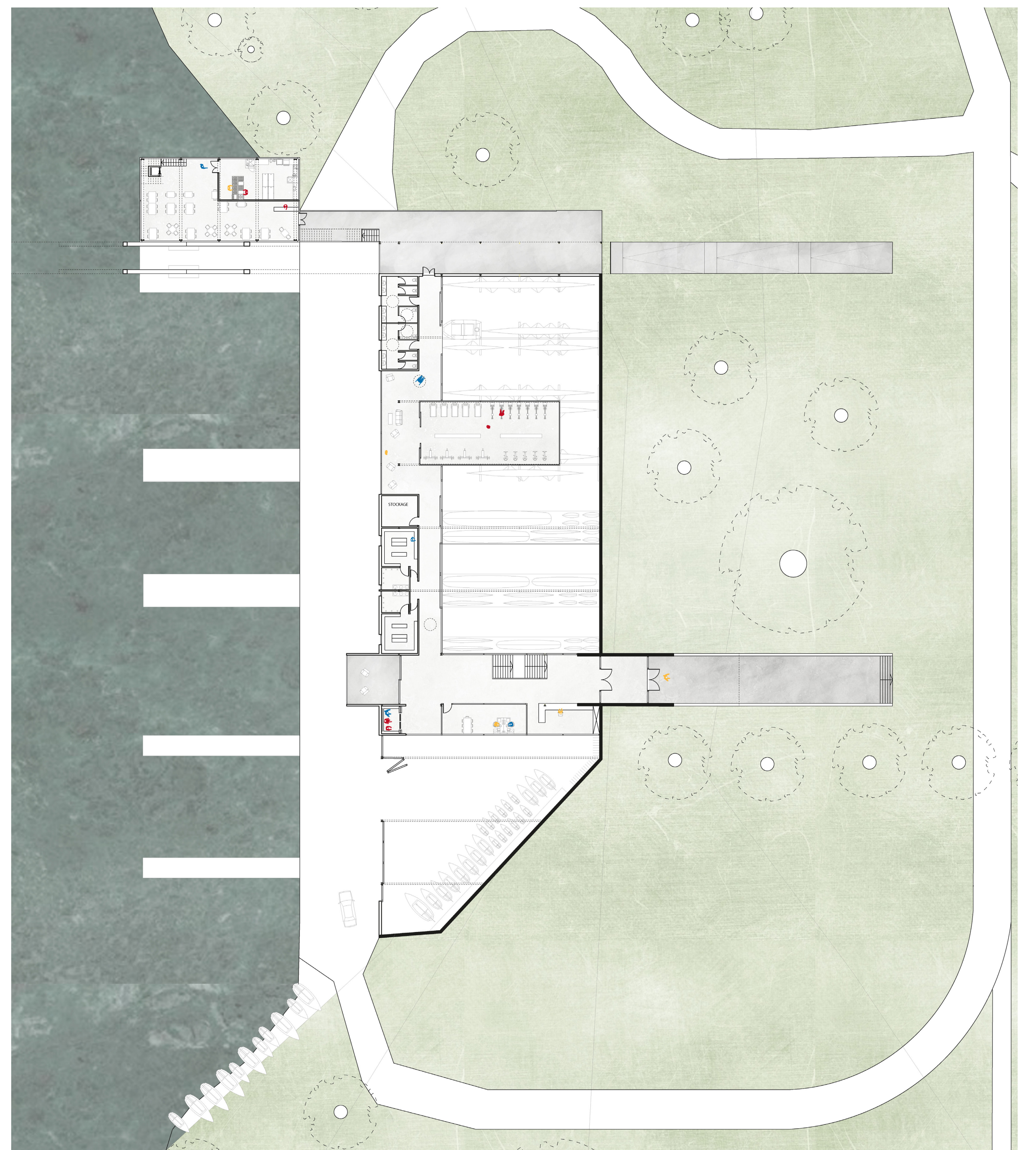
PLAN REZ-DE-CHAUSSEE NIVEAU 0 1/200
