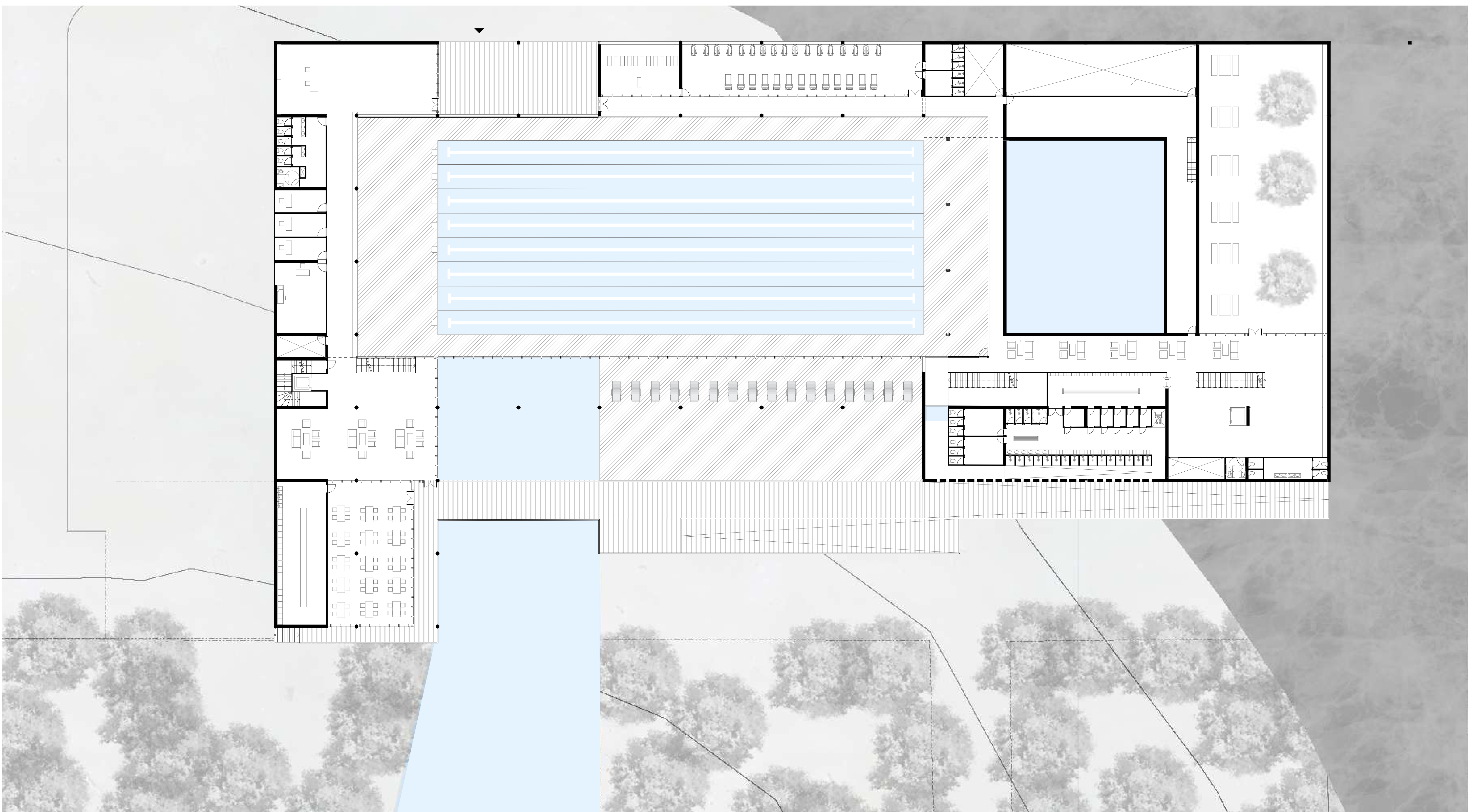
Plan rdc 1:200
