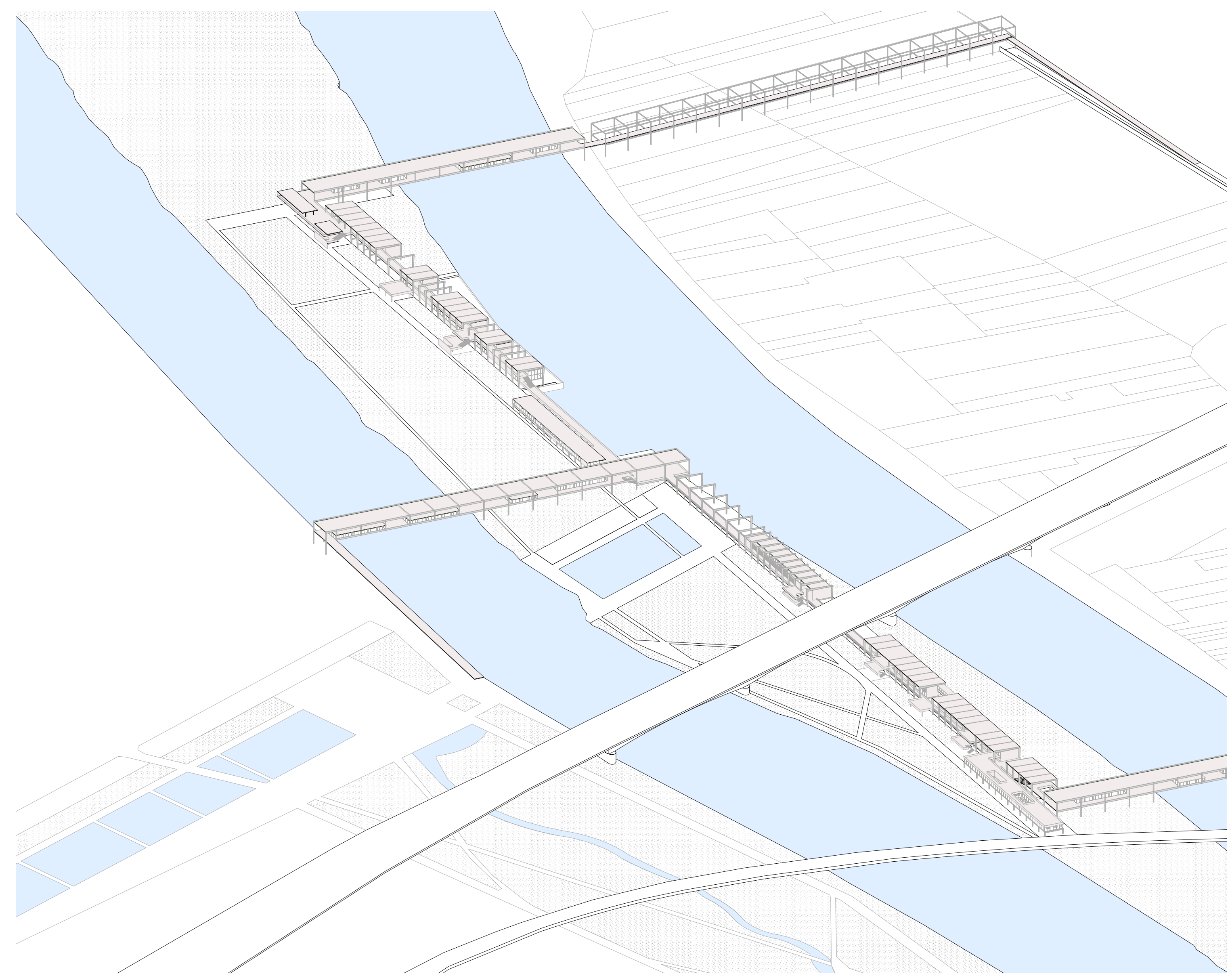
Axonométrie
